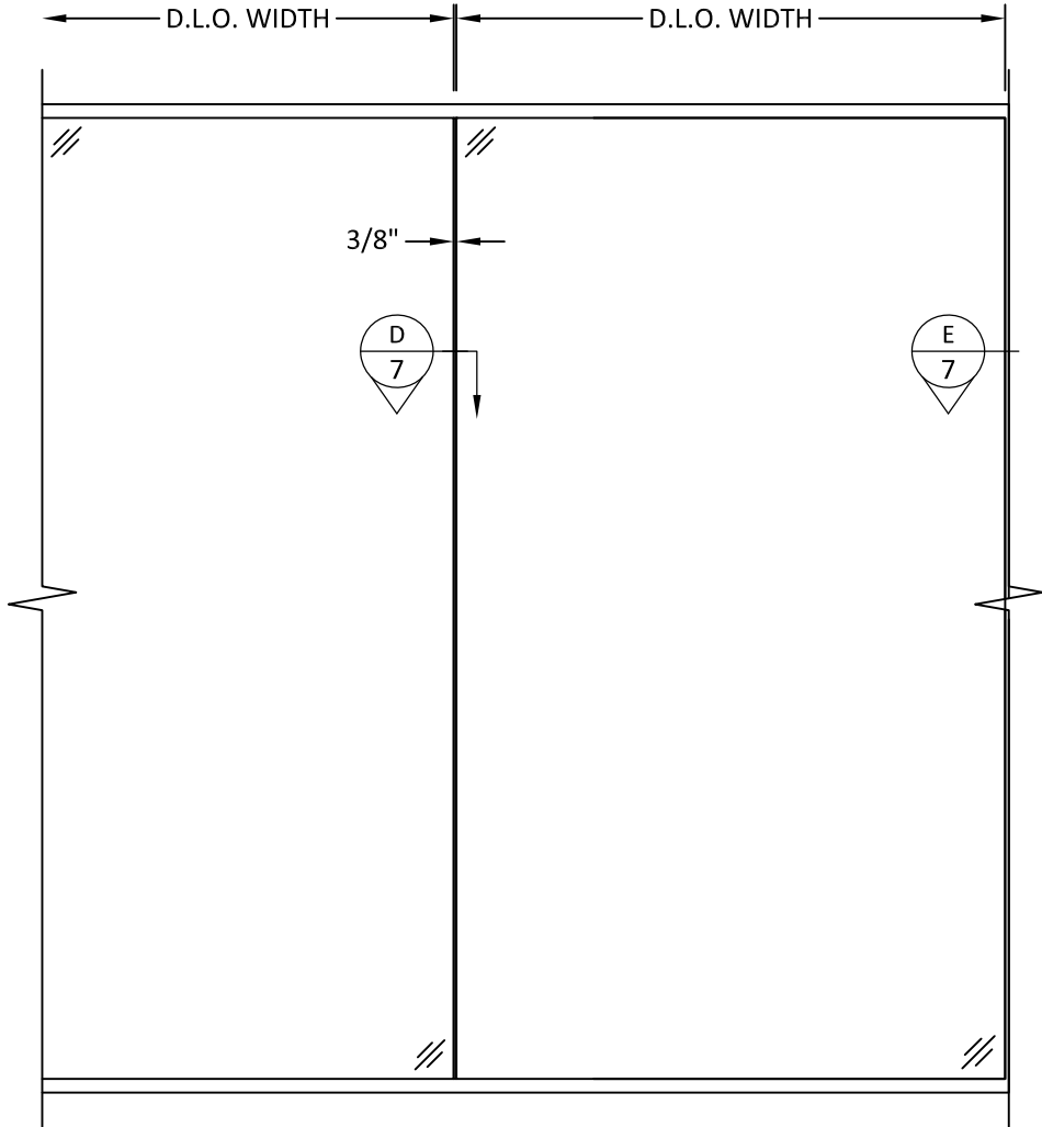
SECTION A-A
